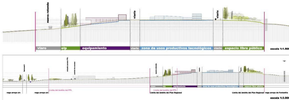
Ilustración 38. Secciones transversales indicativas de la ordenación y su implantación territorial
