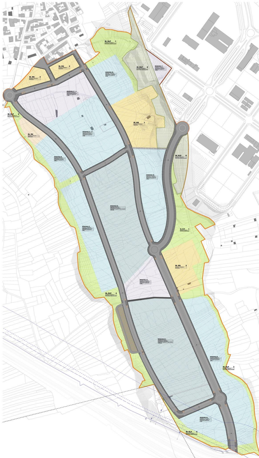
Ilustración 40. Ordenación detallada propuesta para la ampliación del Parque Tecnológico de León
