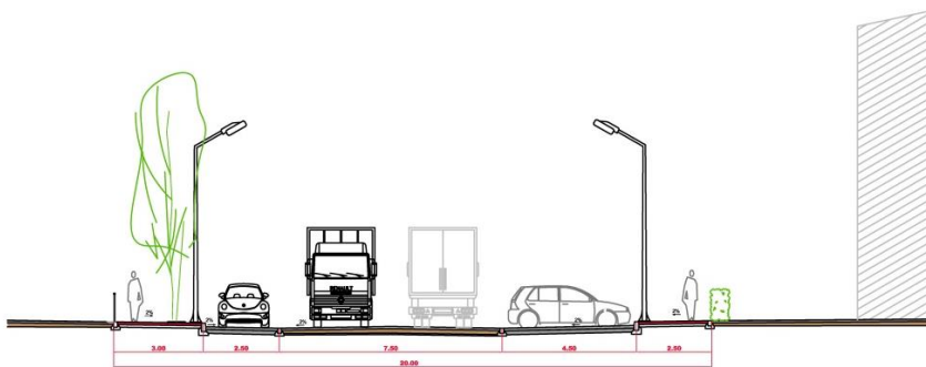
Ilustración 44. Sección tipo de viario de distribución
