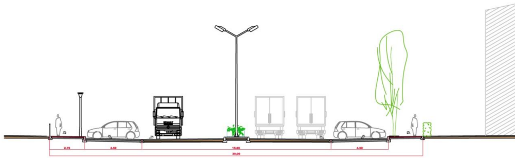
Ilustración 43. Sección tipo de viario estructurante
